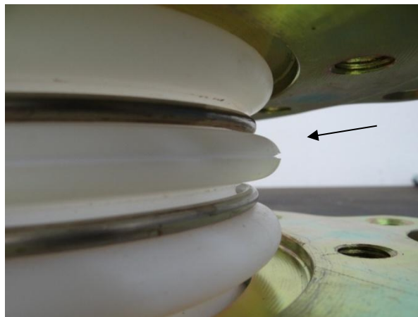
Abb. 7: Rissbildung nach <5000 axialen Bewegungszyklen aufgrund ungleichmäßiger Wandstärkenverteilung
